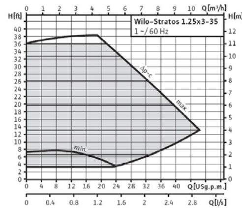
Δp-c (constant)
