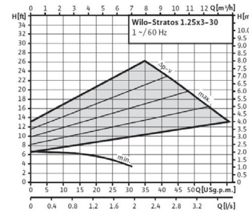
Δp-v (variable)
